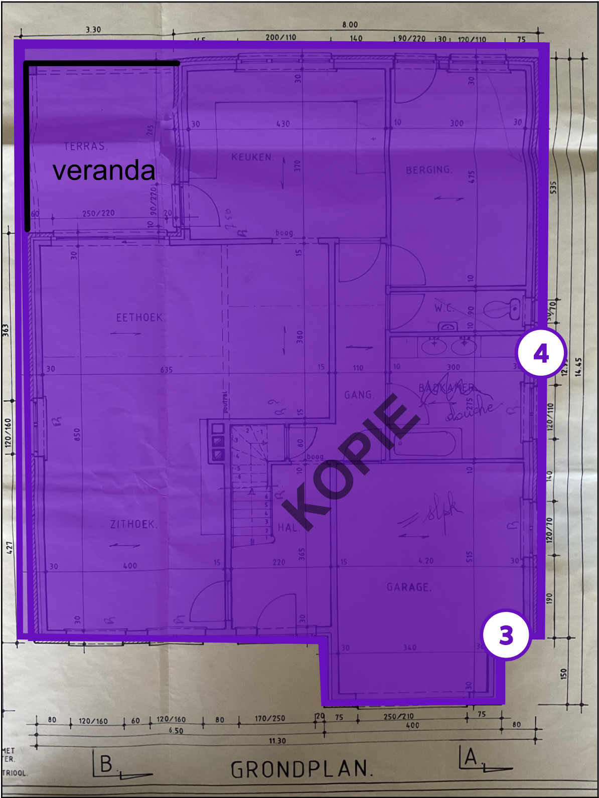
Legende van plan 1.6: Plan van het gelijkvloers
