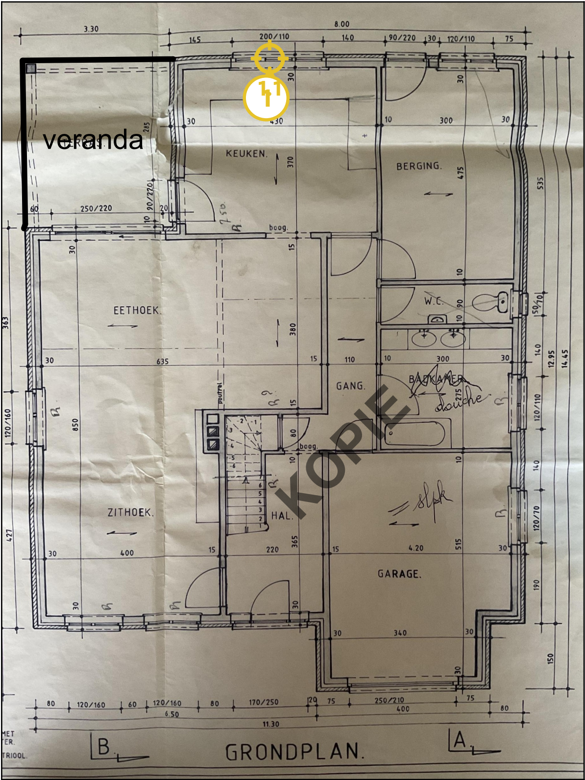
Legende van plan 1.4: Plan van het gelijkvloers
