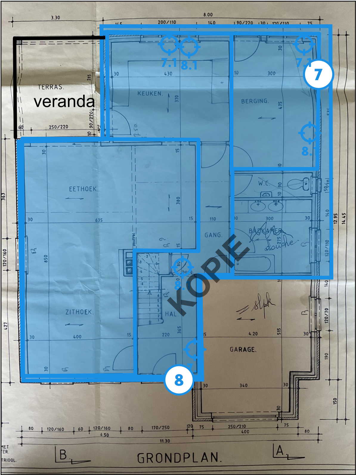
Legende van plan 1.3: Plan van het gelijkvloers
