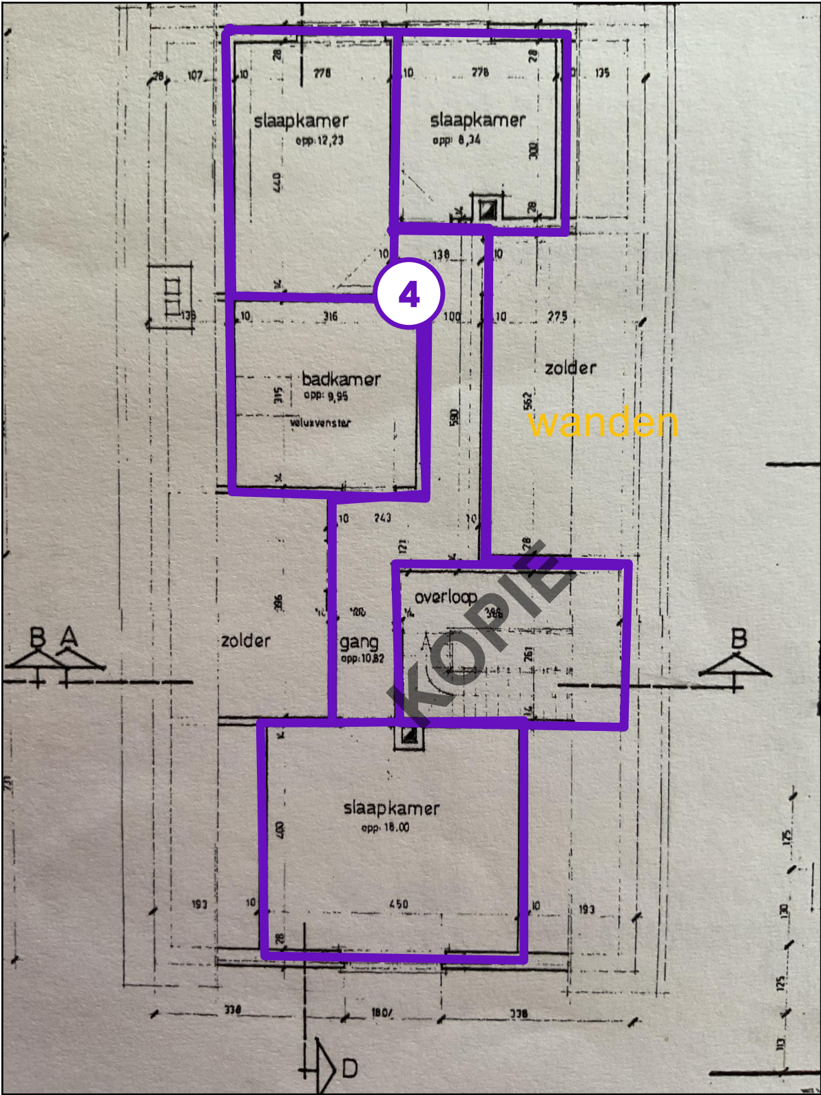
Legende van plan 1.9: Plan van de eerste verdieping
