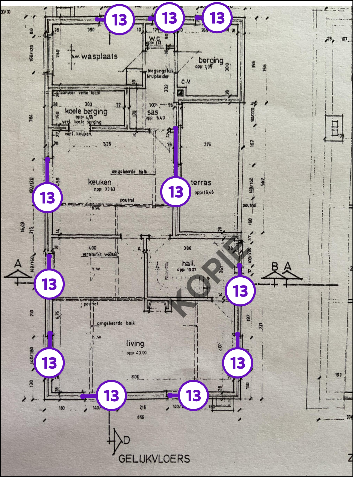
Legende van plan 1.6: Plan van het gelijkvloers
