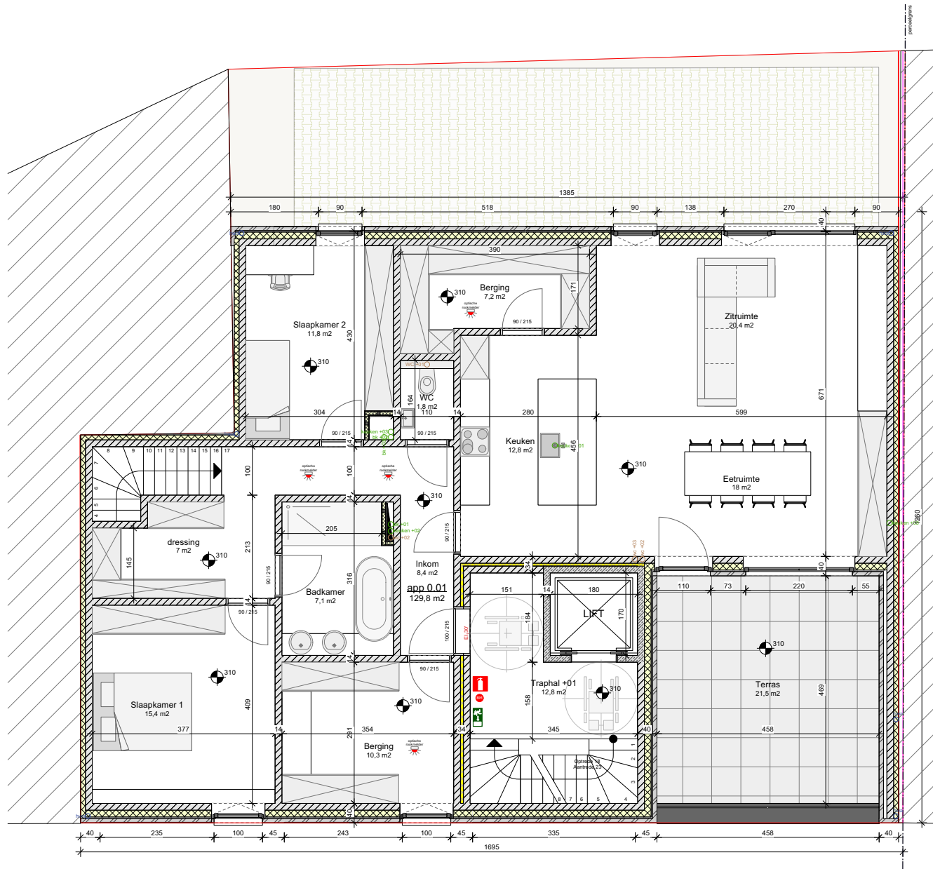
Verdieping +01 1:50
